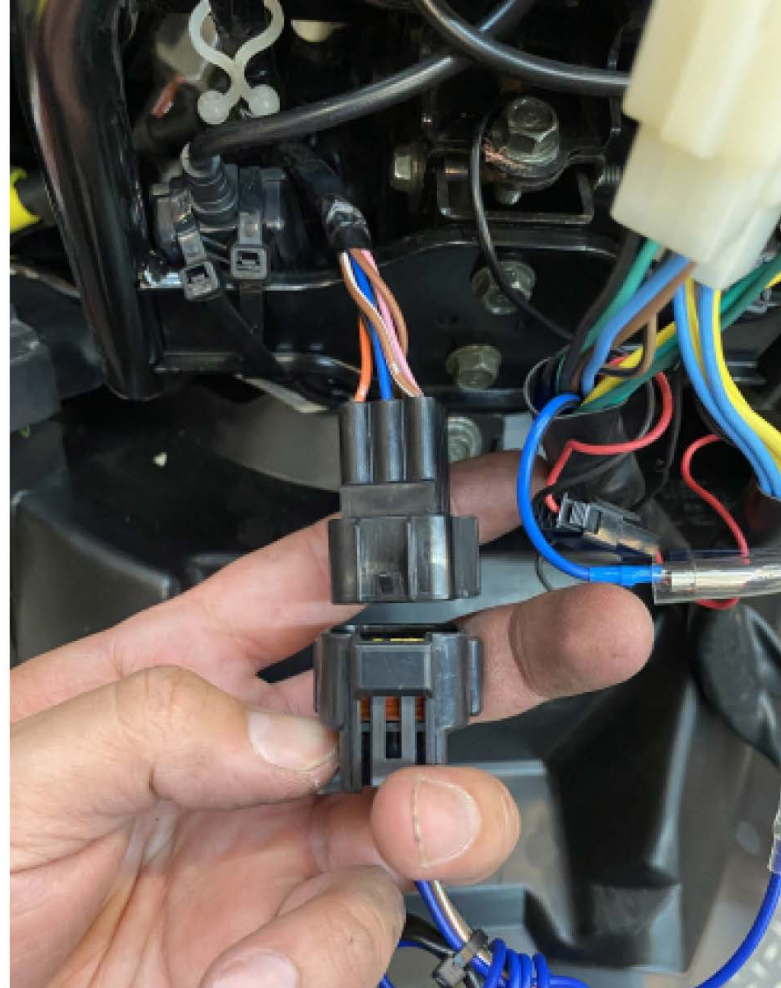
⑨ 將小燈線串聯上去
