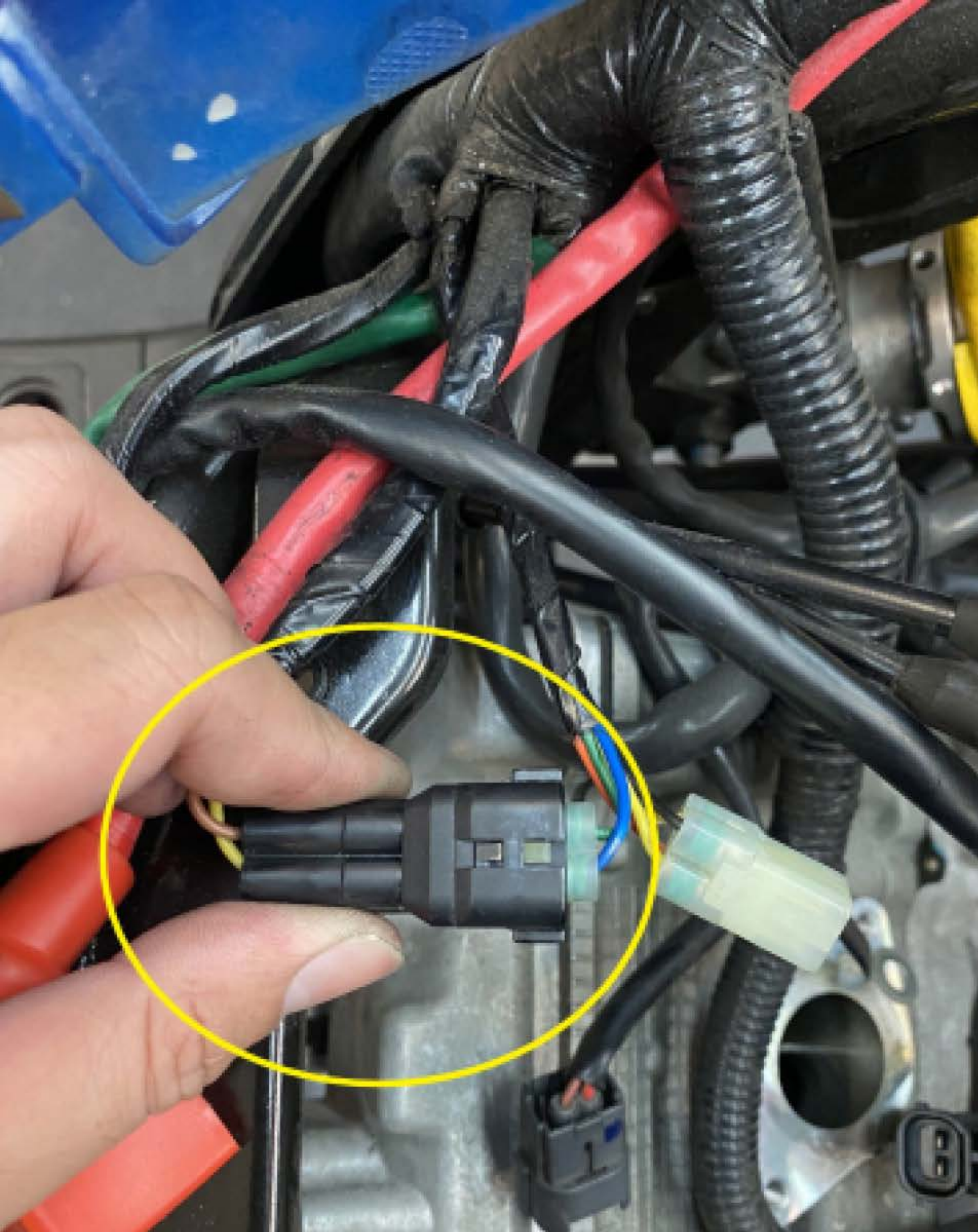
② 找出牌照燈線
