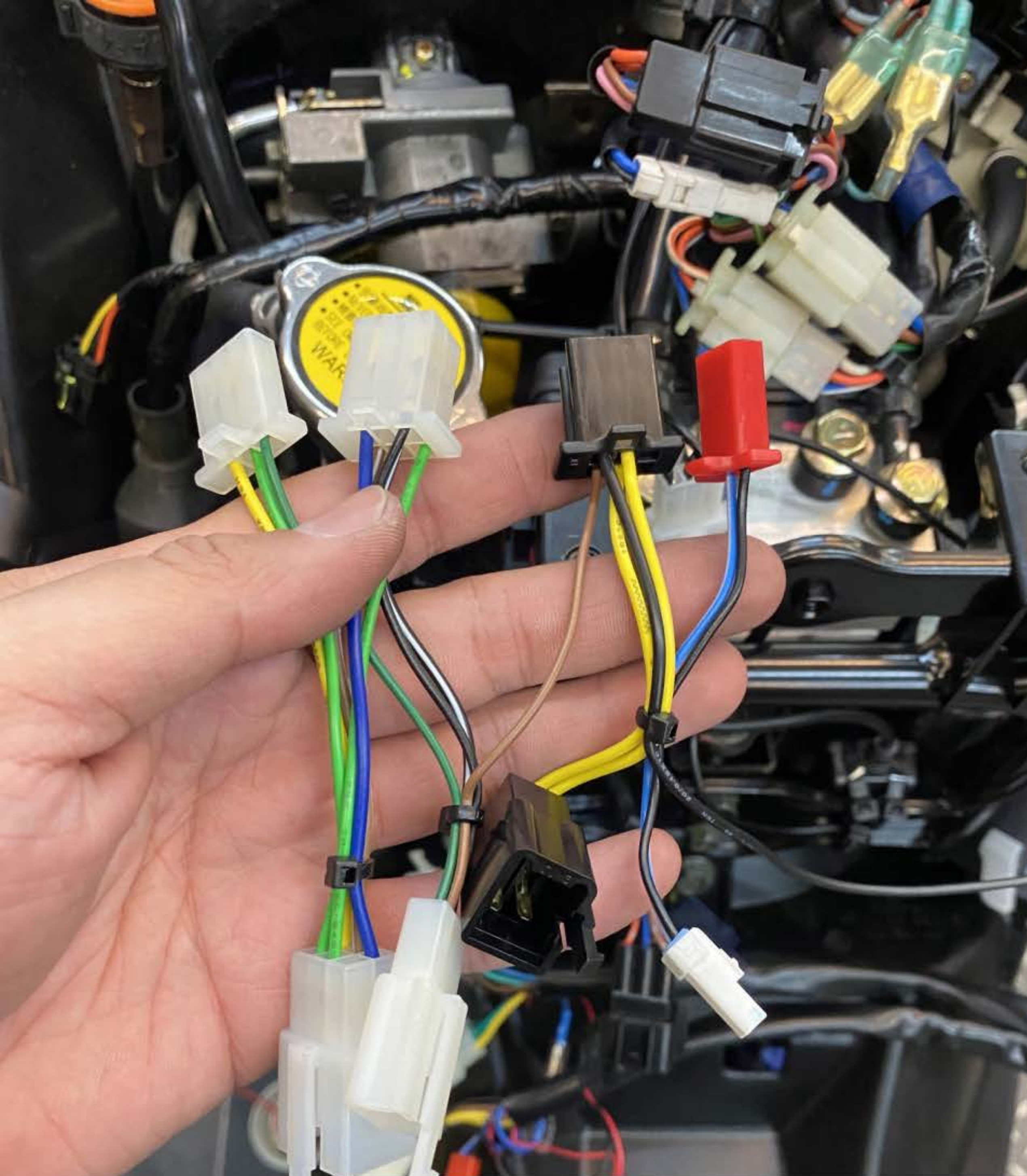
③ 拿出發光開關 專用轉接線
