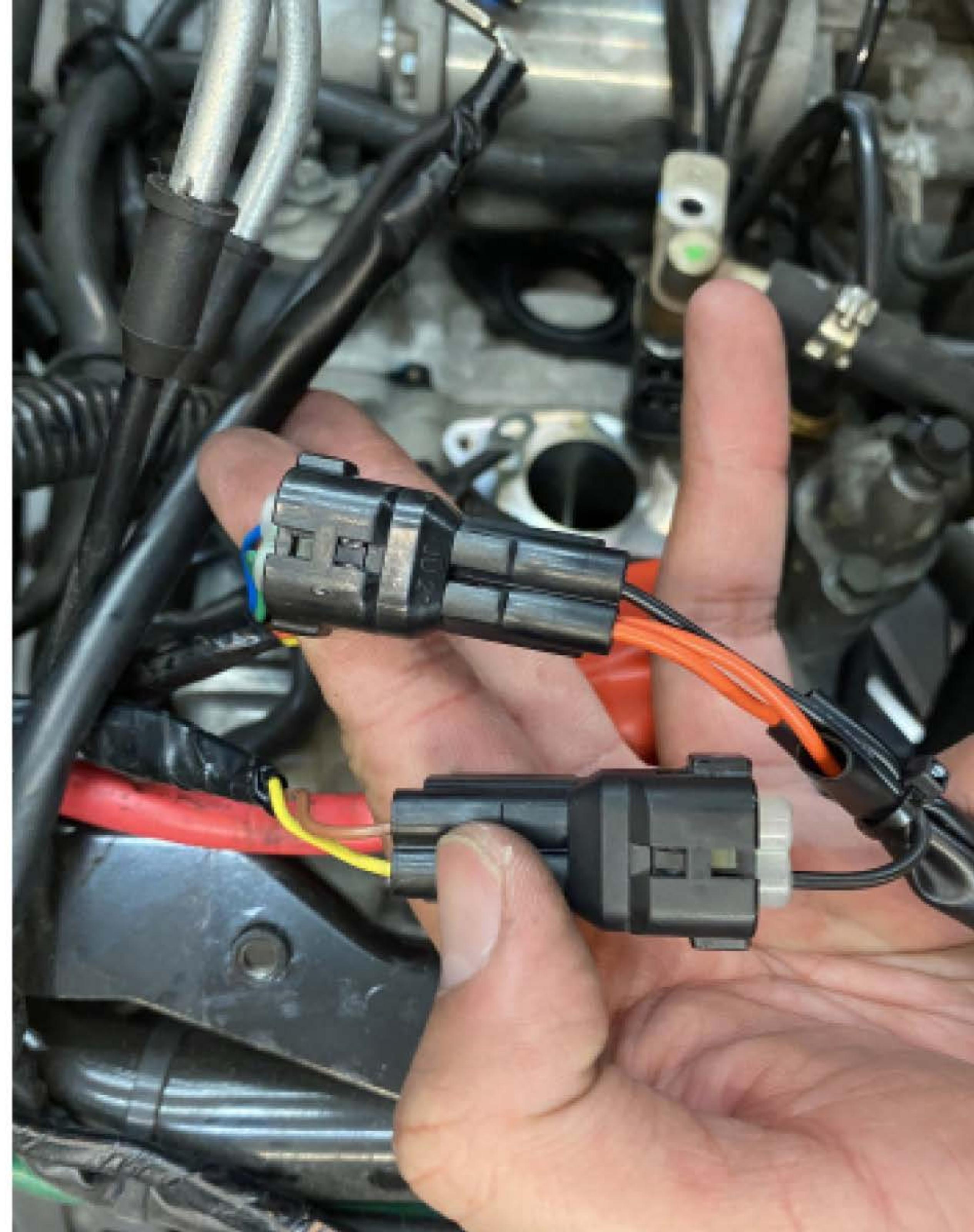
③ 將小燈線與它串接
