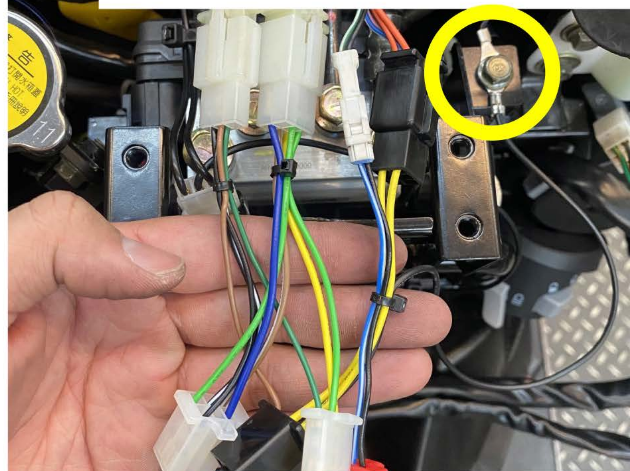
❖ Y 字頭需鎖上車台 (接負電)
